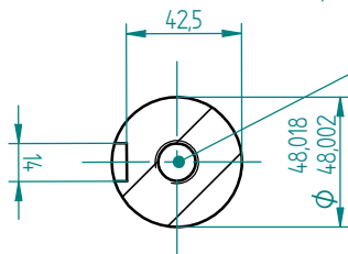
Przekrój A-A 1:2
